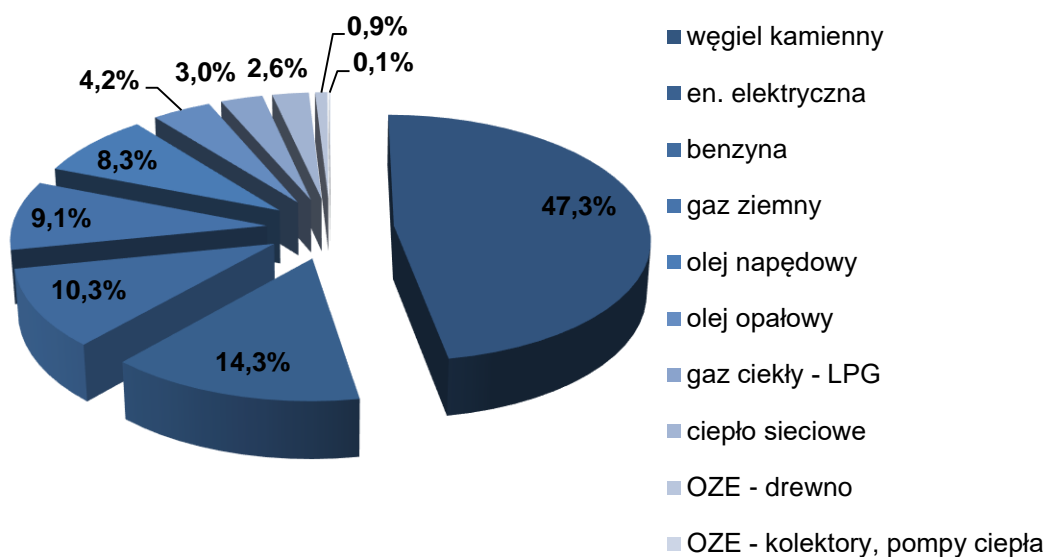
Wykres 27. Udział poszczególnych nośników energii w końcowym zużyciu energii na obszarze Radziejowa
